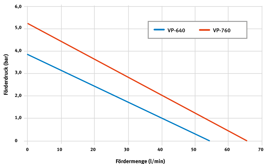
Pumpenkennlinien WT4-90
